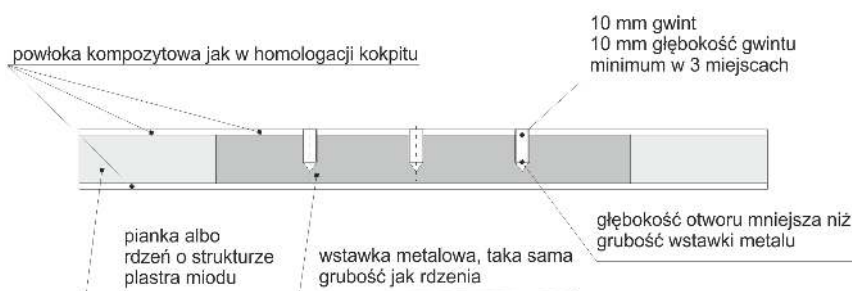
Alternatywne mocowanie zakotwienia pasa pomiędzy nogami zawodnika
